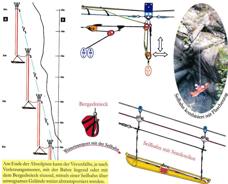
Horizontale Seilbahn kombiniert mit vertikalem Flaschenzug (Kransystem)
